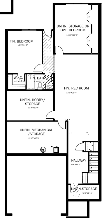
OPTIONAL BASEMENT
